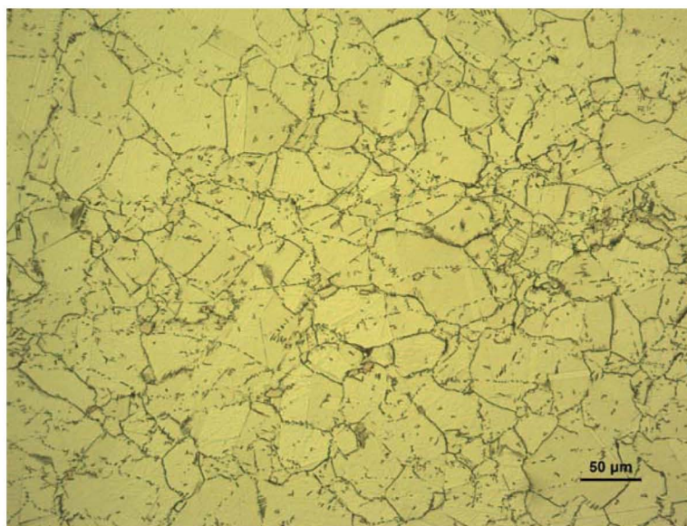
图A.6 a) \delta ( \text{Ni}_3\text{Nb} )相可接受极限照片 (250X)
