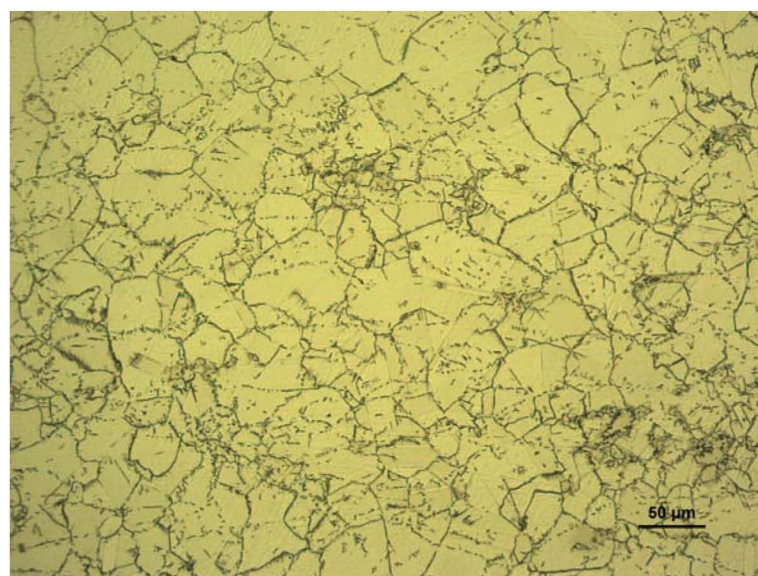
图A.6 b) \delta ( \text{Ni}_3\text{Nb} )相不可接受极限照片 (250X)
